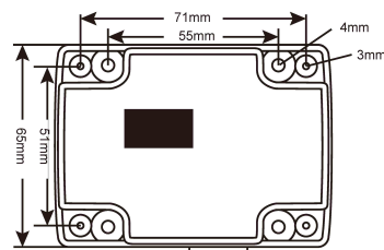
接線盒尺寸圖
