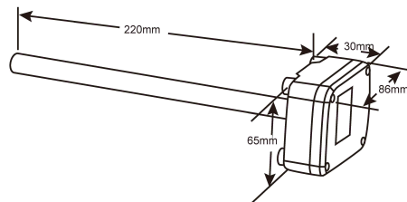
接線盒尺寸圖
