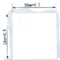
開孔尺寸
