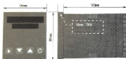
外形尺寸
